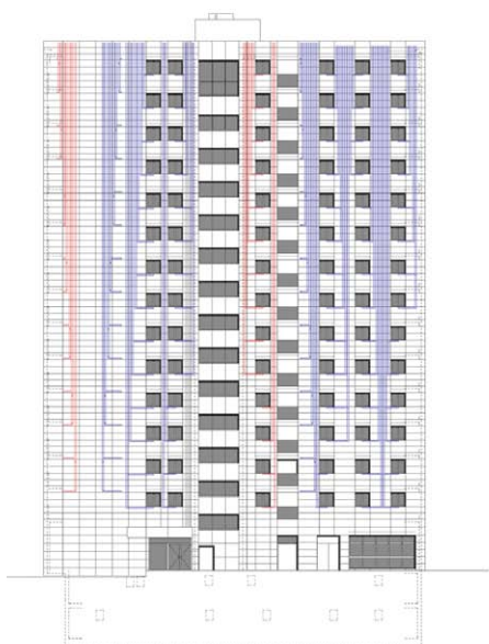
Intégration des canaux de ventilation dans la façade
